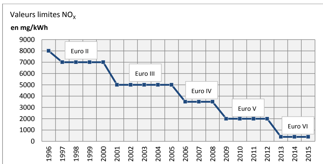
Figure 48: Evolution des valeurs limites d'émissions de \text{NO}_x selon les normes les plus récentes
